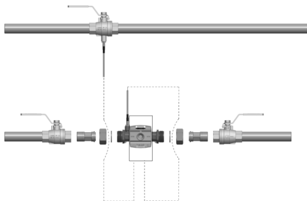
Abb. 2: Beispiel für Einbau mit Kugelhahn und Zähler mit 110 mm Armatur
