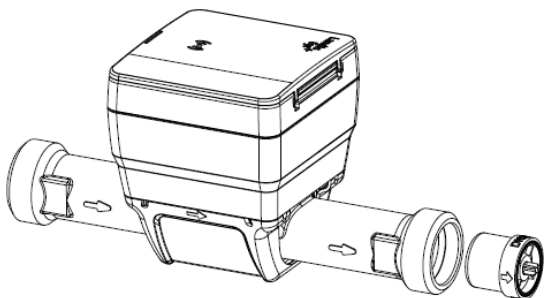
Abbildung 3: Einbau Rückflussverhinderer (als Zubehör erhältlich)
