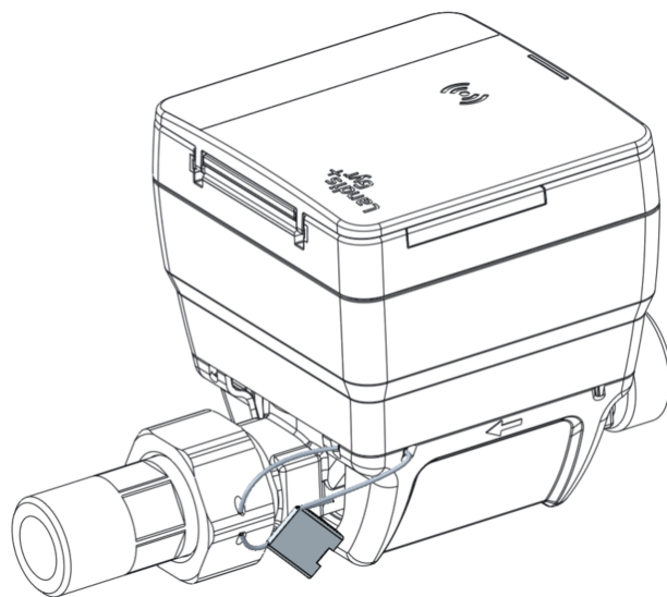
Abbildung 5: Beispiel Verplombung mit Drahtplombe
