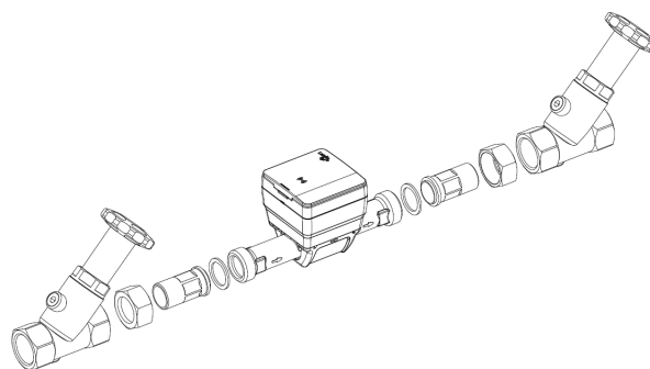
Abbildung 1: Beispiel Einbau
