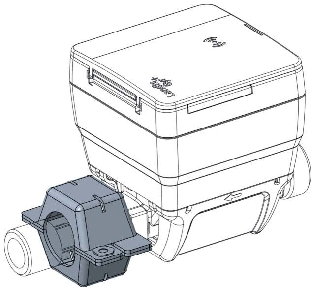
Abbildung 6: Beispieldichtung mit Dichtungsschelle (als Zusatzelement erhältlich)
